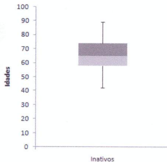
BOXPLOT INATIVOS
